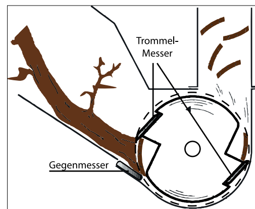
Trommelhackwerk
