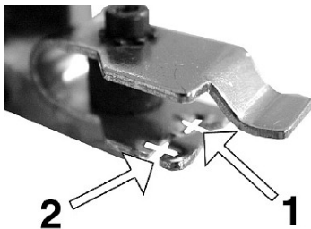
Abb. 12: Sägeblatt einsetzen
