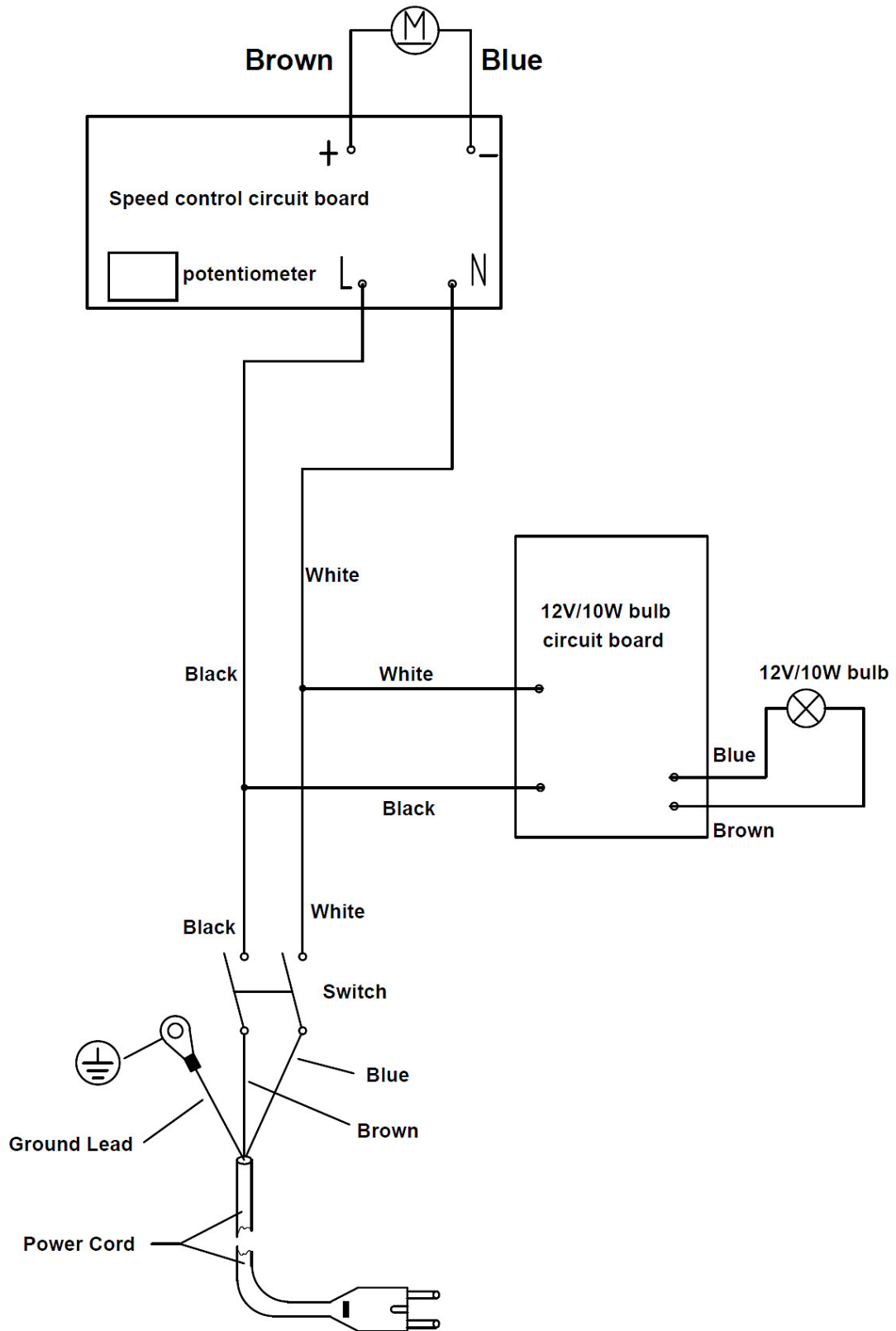
Abb. 27: Elektro-Schaltplan DKS 504 Vario
