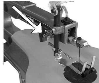
Abb. 14: Werkstückniederhalter positionieren
