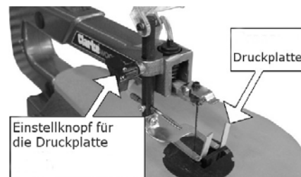
Abb. 17: Abblasvorrichtung einstellen
