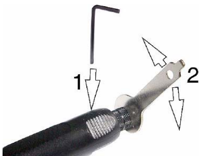
Abb. 22: Werkzeug wechseln
