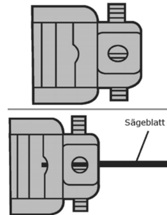
Abb. 5: Sägeblattadapter einsetzen
