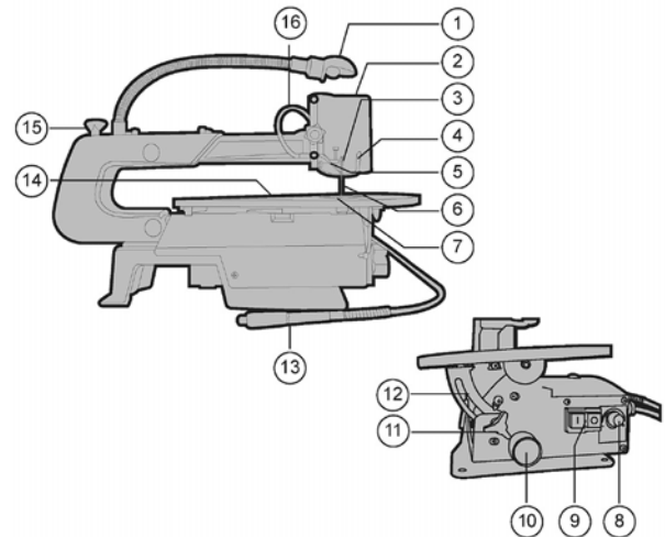
Abb. 3: Dekupiersäge
