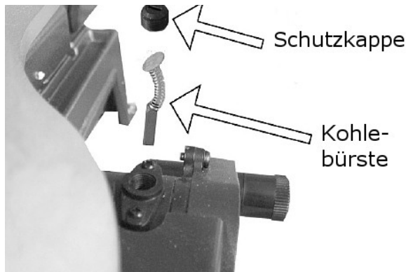
Abb. 23: Kohlebürsten wechseln
