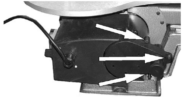
Abb. 24: Riemenabdeckung demontieren
