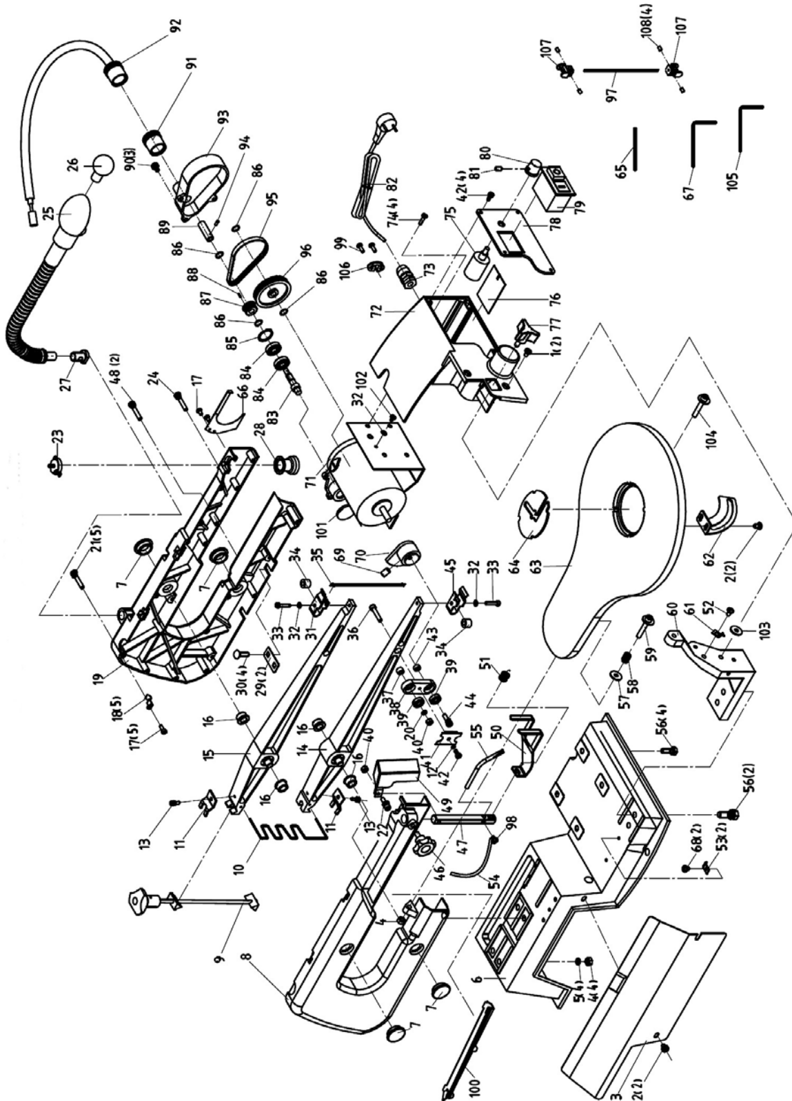
Abb. 26: Ersatzteilzeichnung 1 Dekupiersäge DKS 504 Vario
