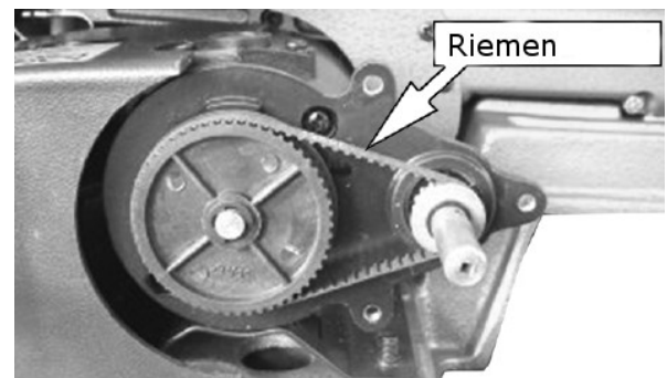
Abb. 25: Antriebsriemen wechseln
