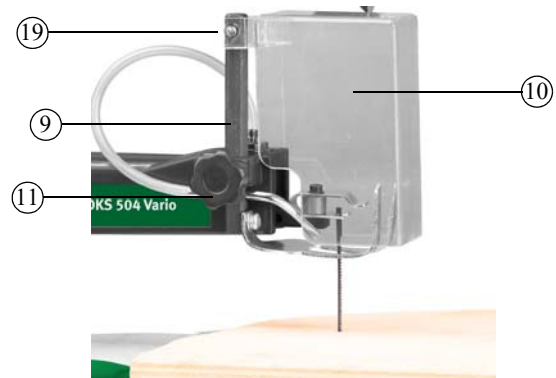
Abb. 9: Montage Sägeblattschutz
