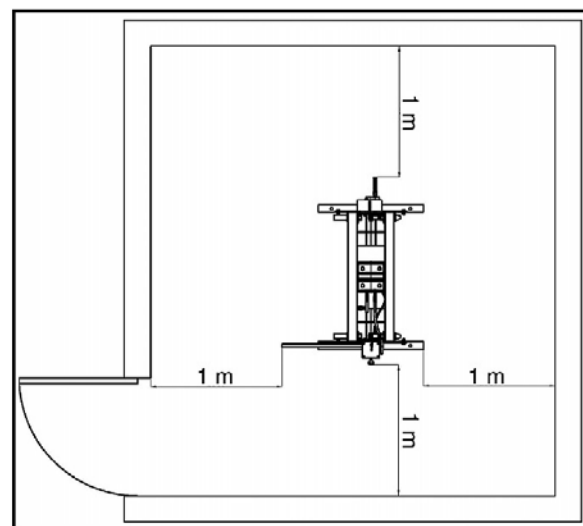
Abb. 6: Korrektes Aufstellen der hydraulischen Werkstattpresse
