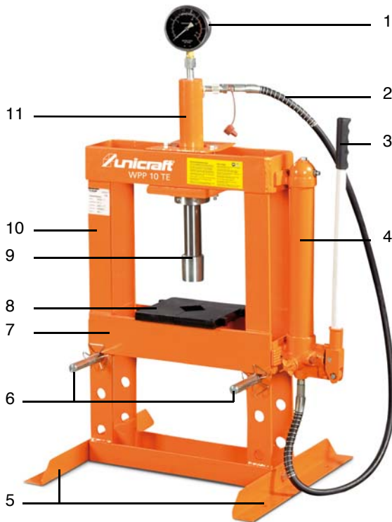
Abb. 5: Hydraulische Werkstattpresse WPP 10 TE
