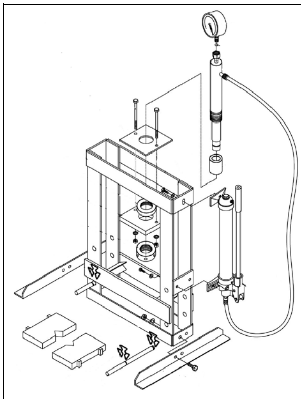
Abb. 7: Zu montierende Teile der hydr. Werkstattpresse WPP 10 TE
