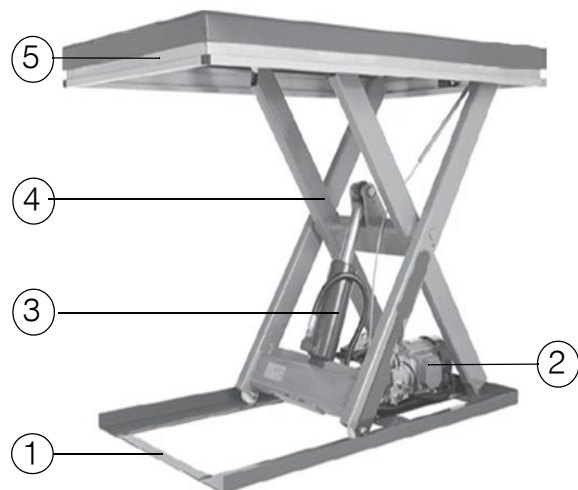
Abb. 2: Gerätebeschreibung
