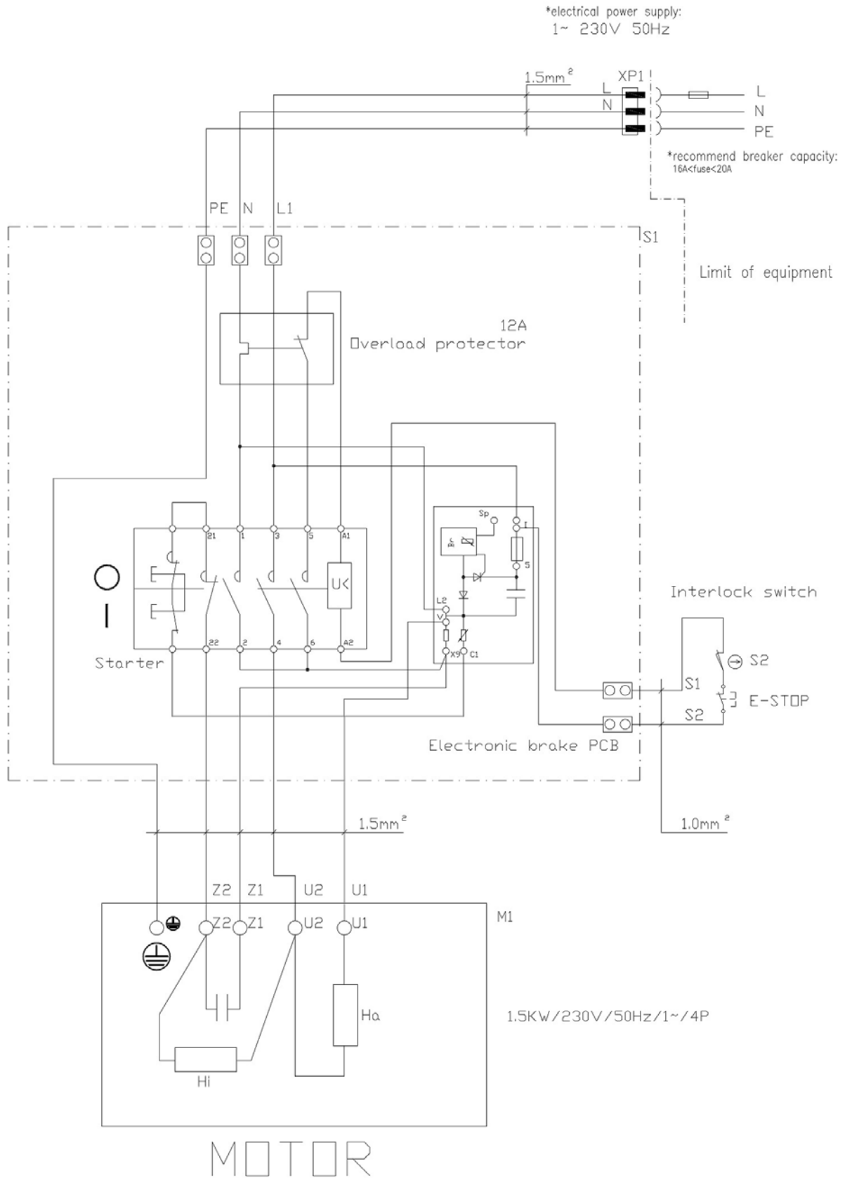
Abb. 26: Elektro-Schaltplan Holzbandsäge HBS 431
