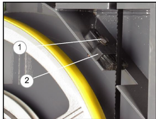
Abb. 14: Spänebürste
