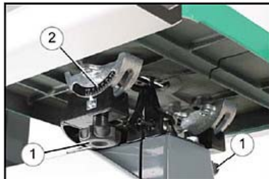
Abb. 7: Schwenken des Arbeitstisches. Unten: Modell HBS 351
