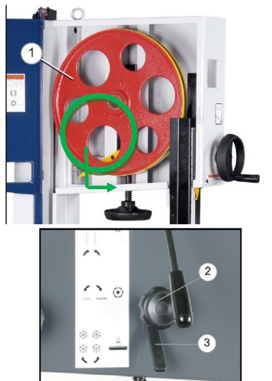
Abb. 12: Einstellen des Sägebandlauf
