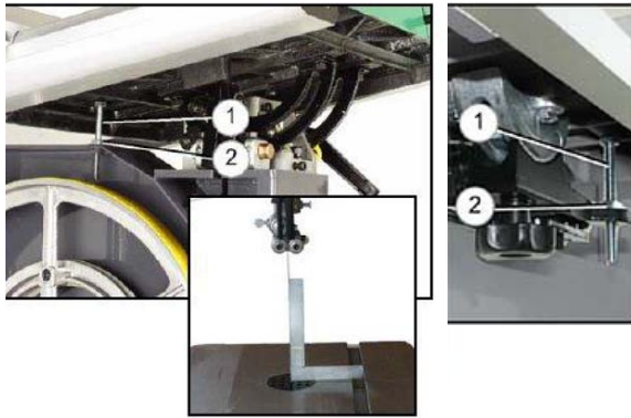
Abb. 8: 0° Stellung Arbeitstisch. Rechts: Modell HBS 351
