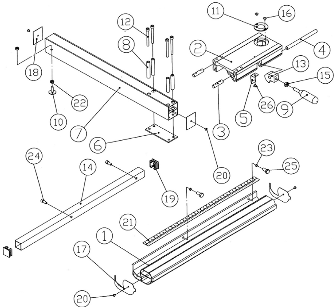
Abb. 22: Ersatzteilzeichnung 3 HBS 533
