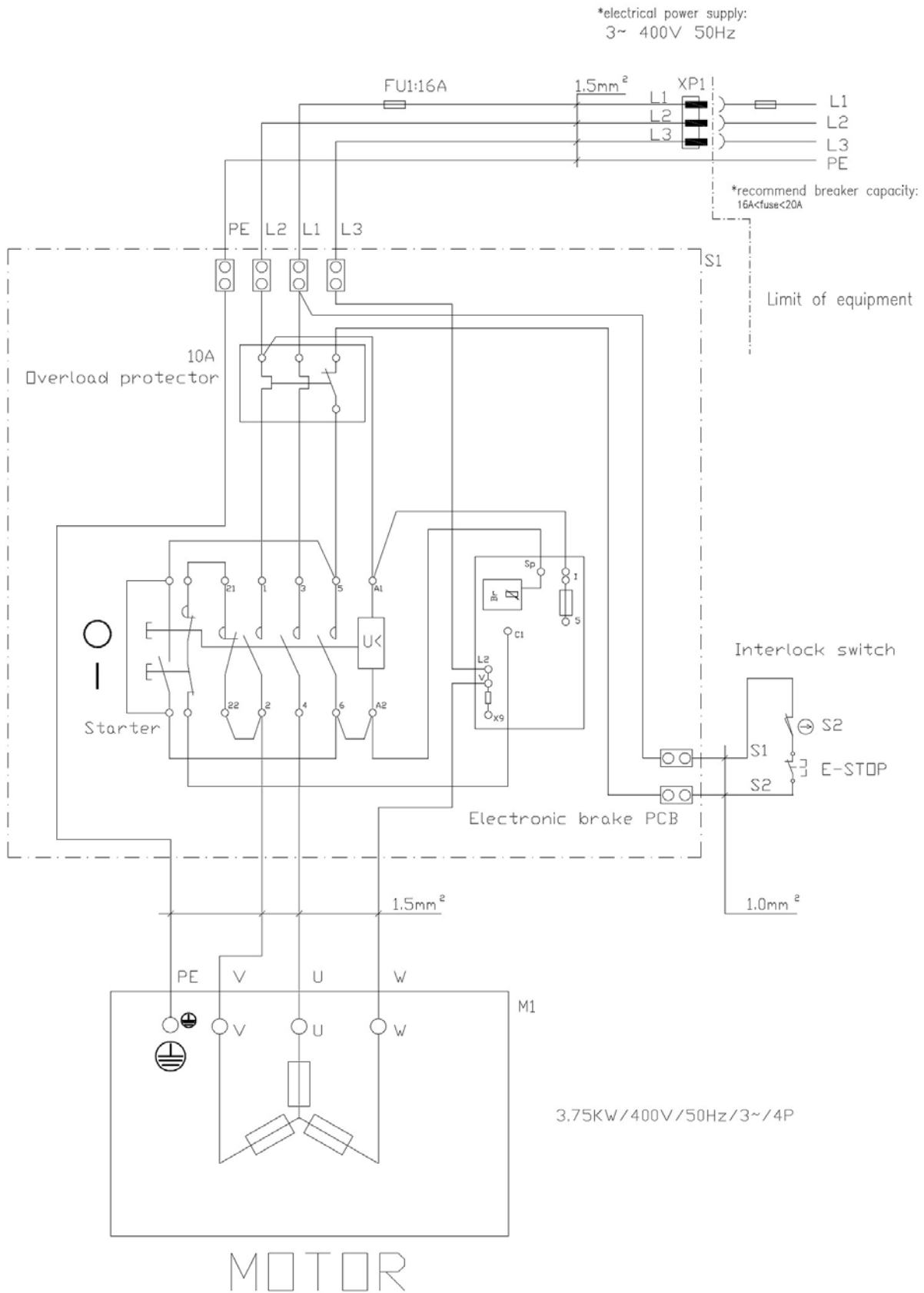
Abb. 27: Elektro-Schaltplan Holzbandsäge HBS 433 und HBS 533
