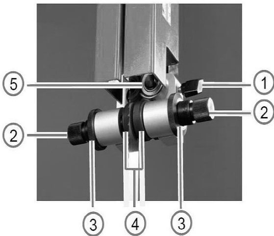
Abb. 13: Einstellen der Sägeblattführung
