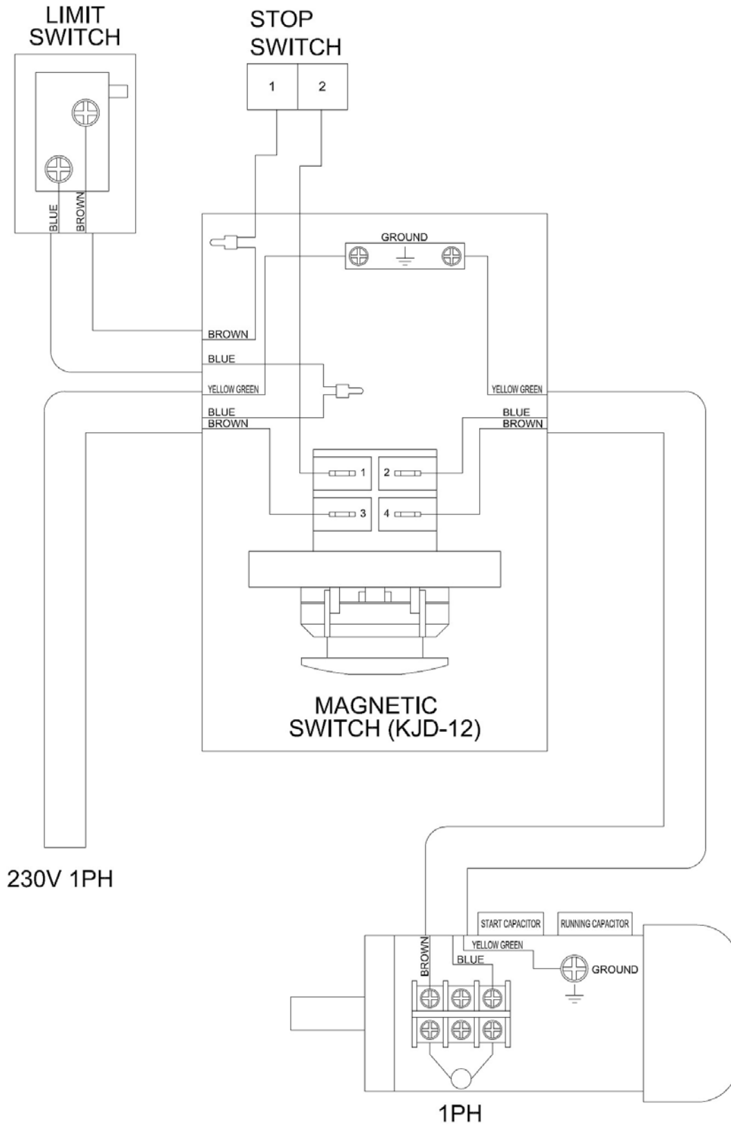
Abb. 25: Elektro-Schaltplan Holzbandsäge HBS 351
