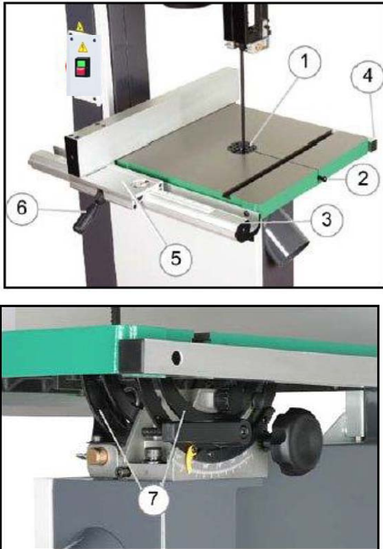
Abb. 5: Montage Bandsäge
