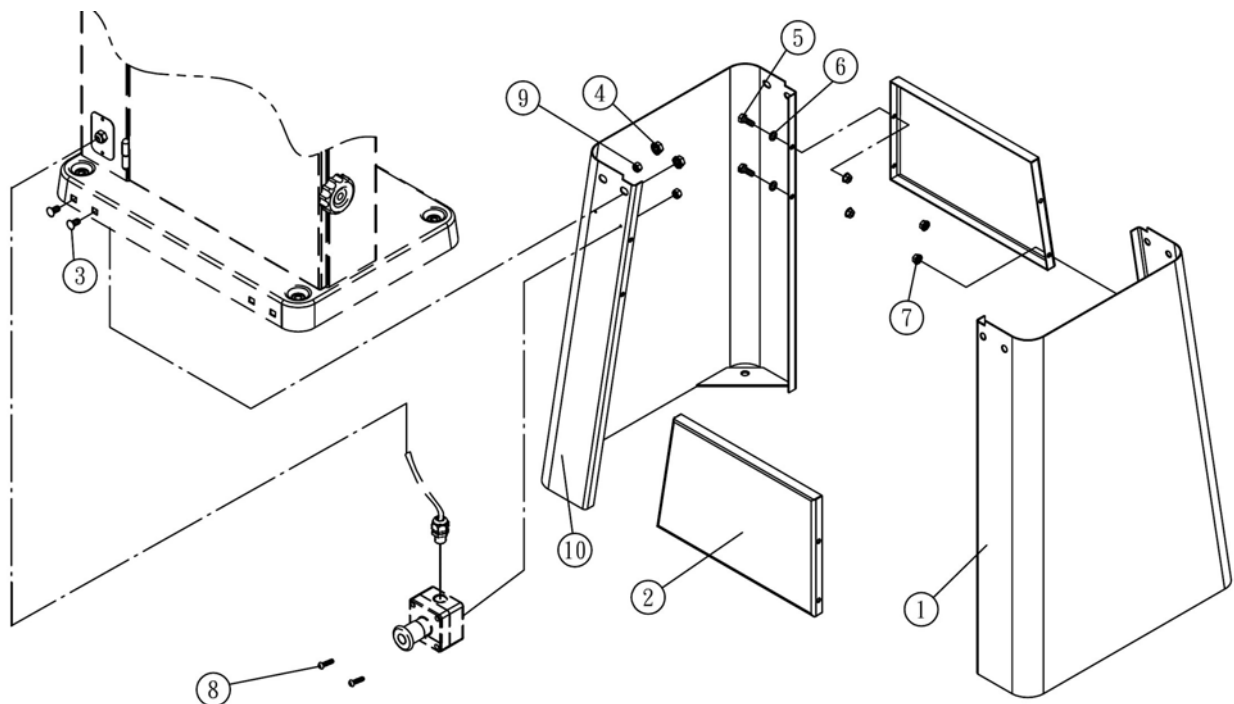
Abb. 24: Ersatzteilzeichnung 2 HBS 351 (oben), Ersatzteilzeichnung 3: Unterbau HBS 351 (unten)
