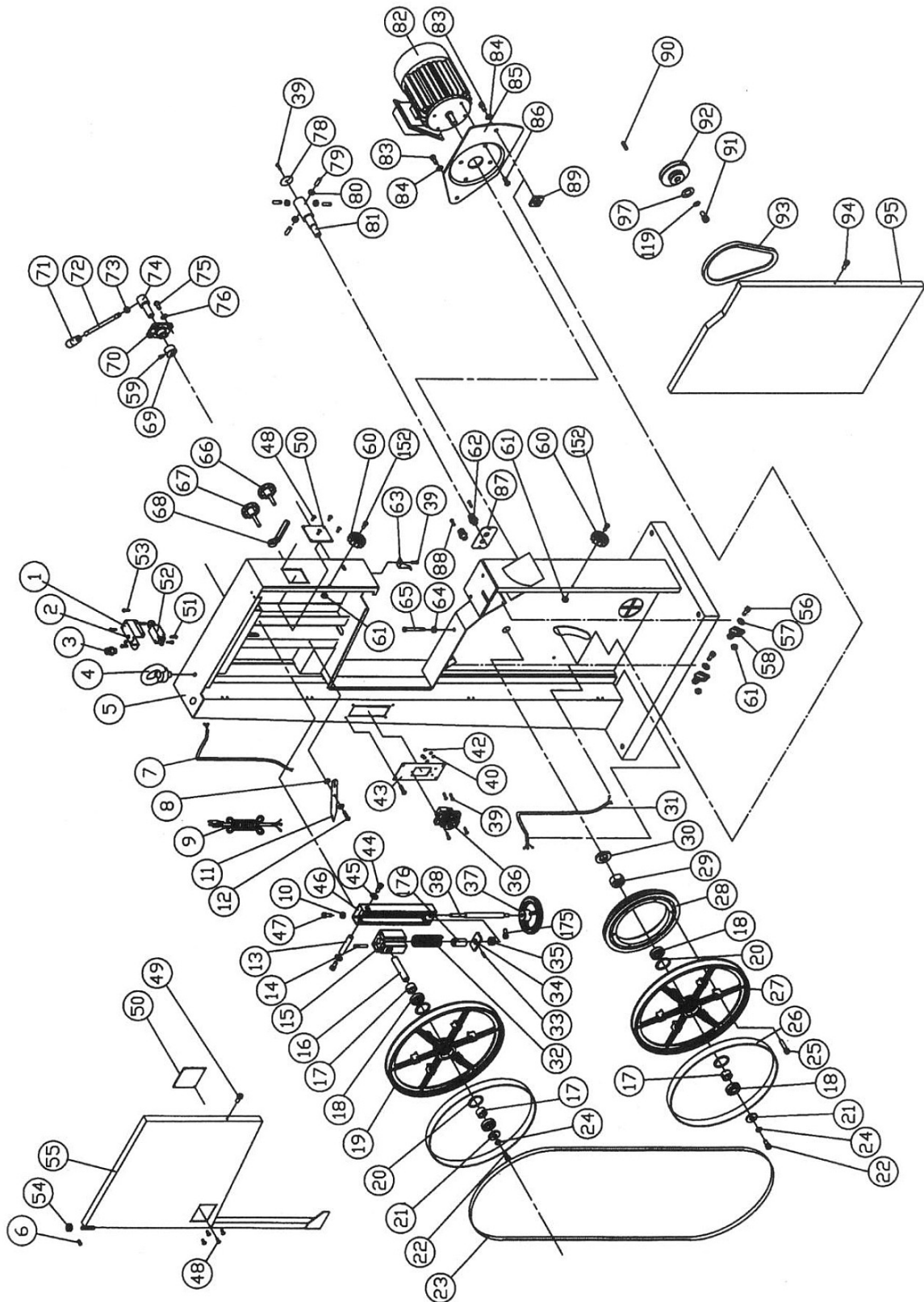
Abb. 20: Ersatzteilzeichnung 1 HBS 533
