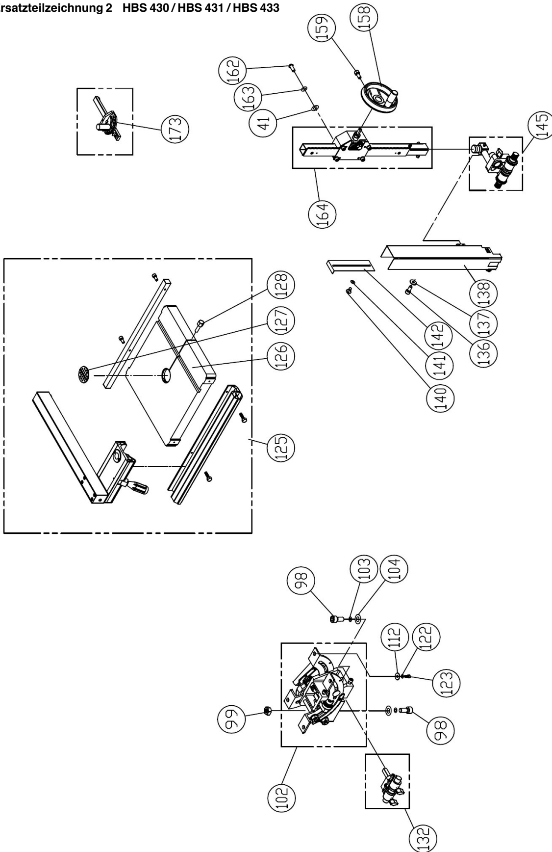
Abb. 19: Ersatzteilzeichnung 2 HBS 430 / HBS 431 / HBS 433
