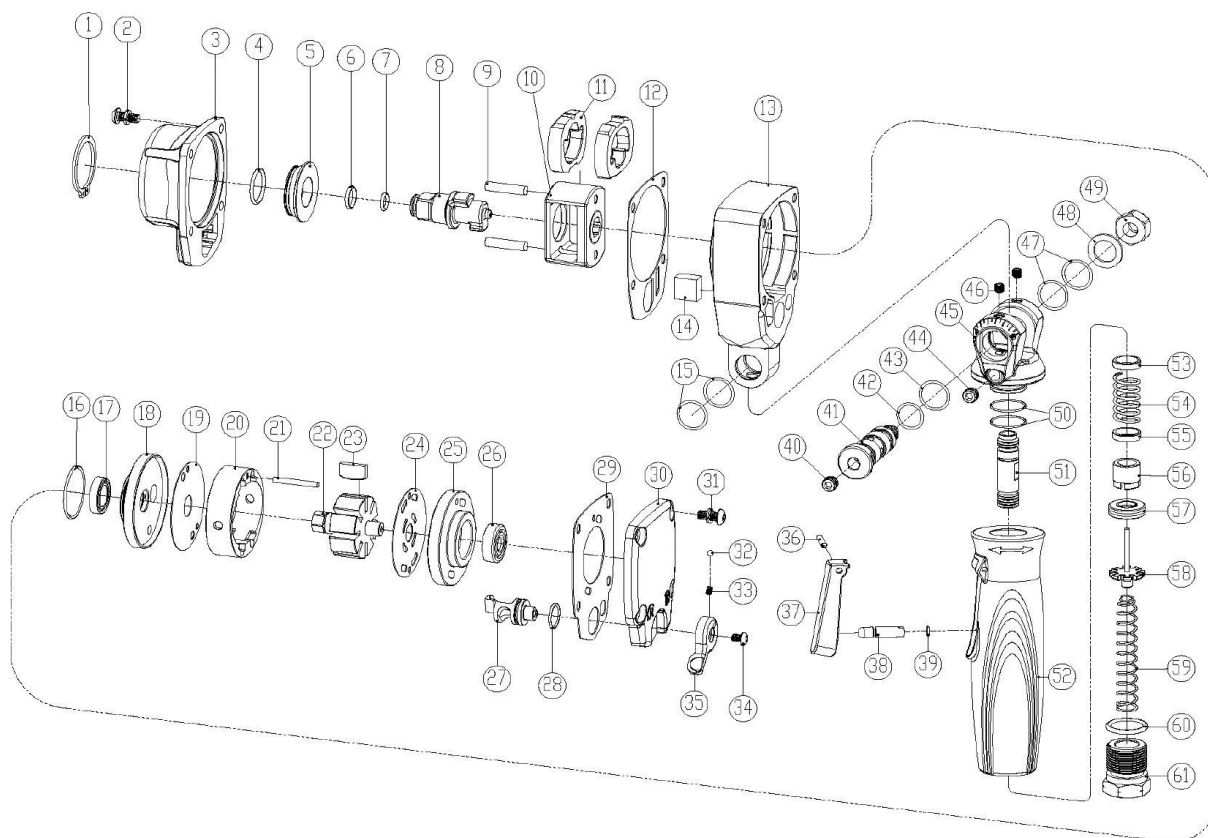
Abb. 3: Ersatzteilzeichnung ISS-TTM 1/2"
