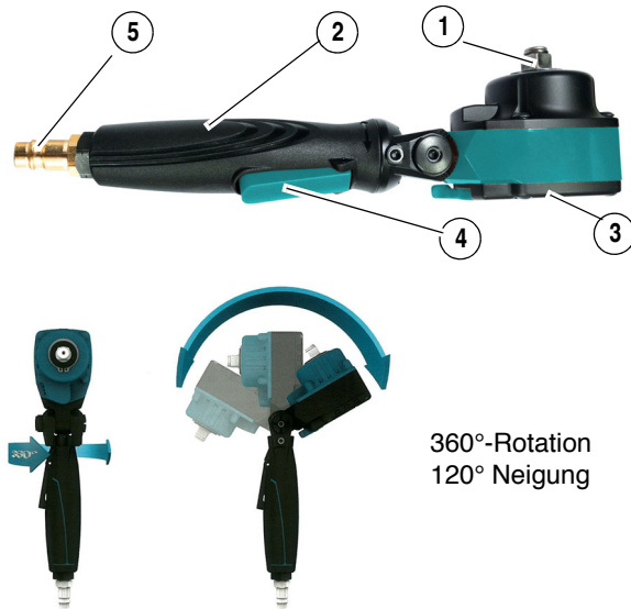
Abb. 2: Bedienelemente ISS-TTM 1/2"
