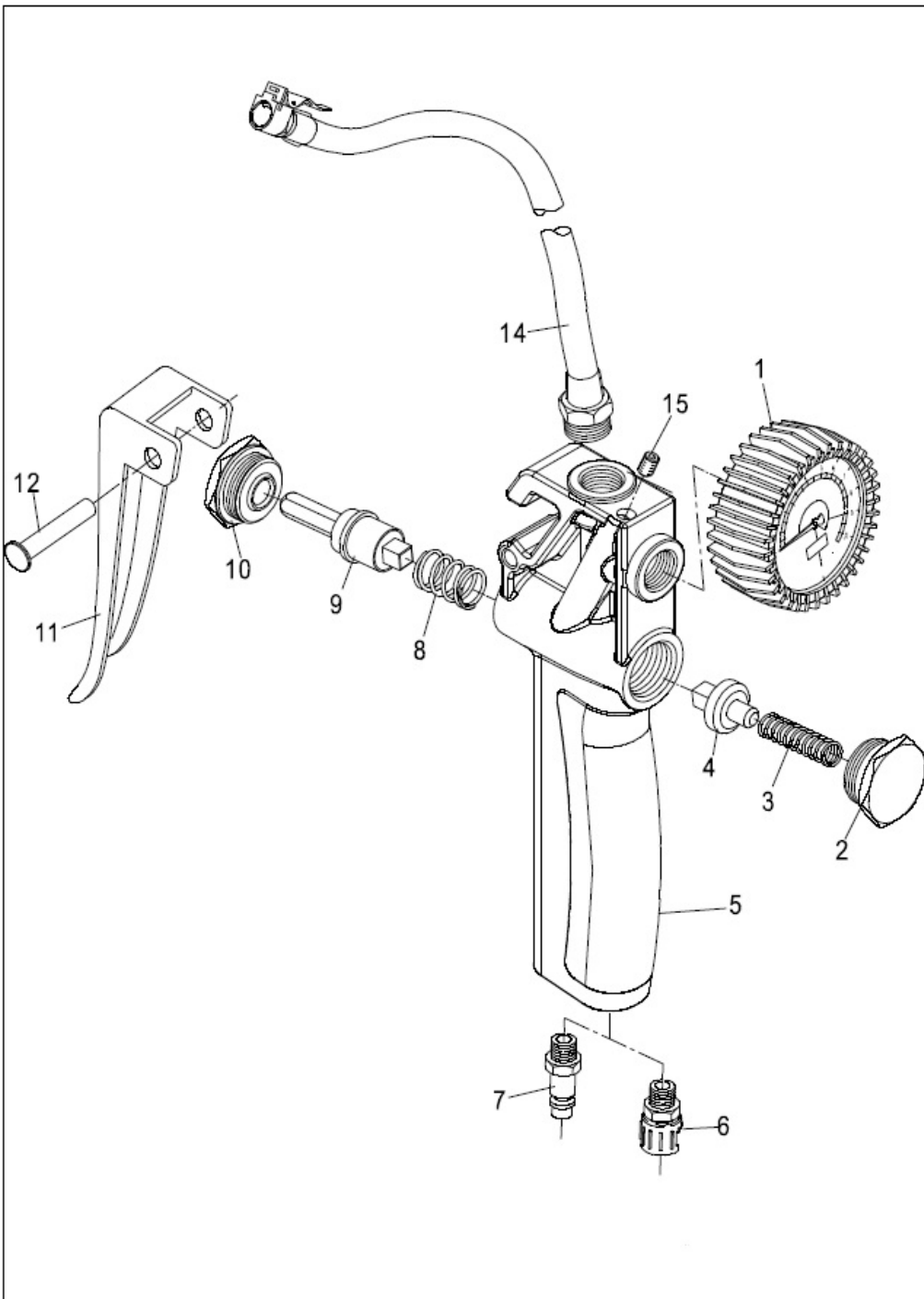
Abb. 2: Ersatzteilzeichnung PRO-G
